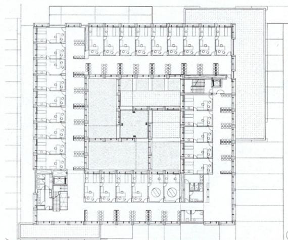
13 · PLANTA PRIMERA
